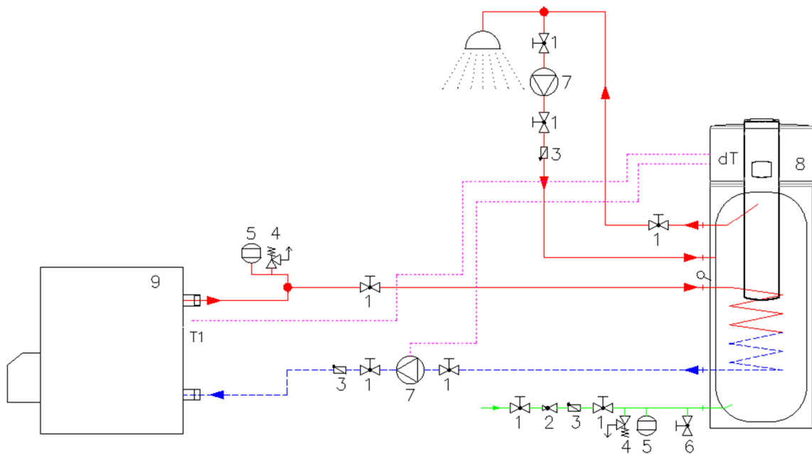
Bild 7: Gerät in Kombination mit Warmwasserspeicher
