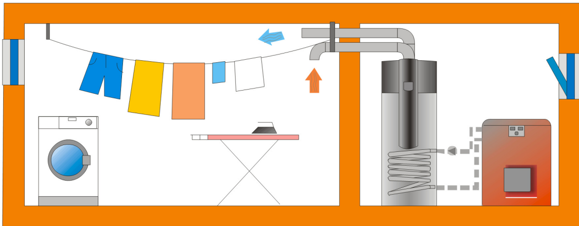
Bild 1: Ansaugen aus dem Nebenraum - Ausblasen in den selben Nebenraum (Nebenumlaufung)
